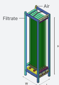
5 Module Skid
