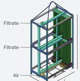
92 Module Skid
