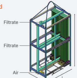
100 Module Skid
